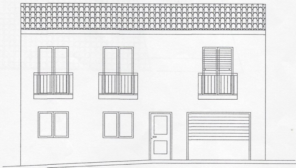
PROSPETTO NORD (progetto di massima)
