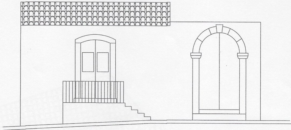
PROSPETTO NORD (stato di fatto)
